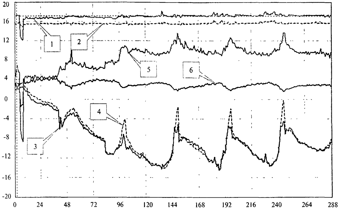
Рис.3. Графики регистрируемых величин, по оси абсцисс отложены точки измерения с интервалом 30 мин. по оси ординат — температура (°С), плотность теплового потока (Вт/м 2 ), сопротивление теплопередаче (м 2 ·°С/Вт)
